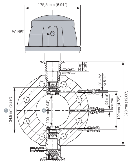
Beispielinstallation einer Flanschzellenadaption für GPro 500.
