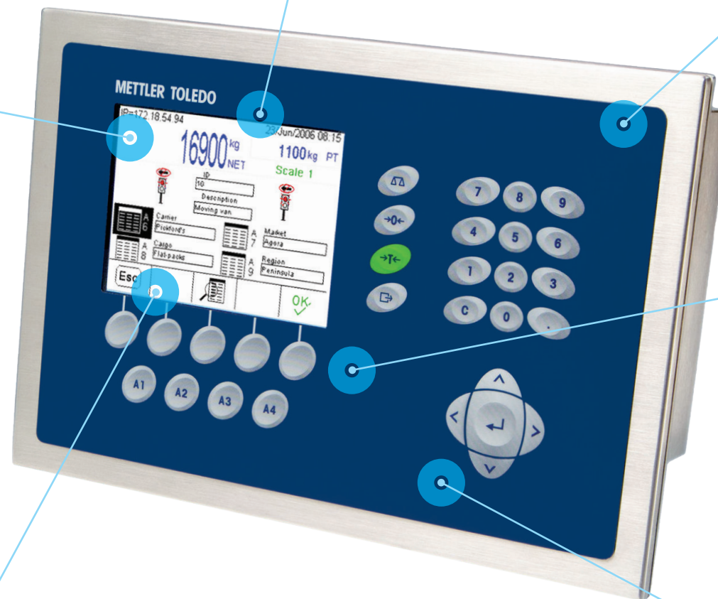
IND780 계량 인디케이터
