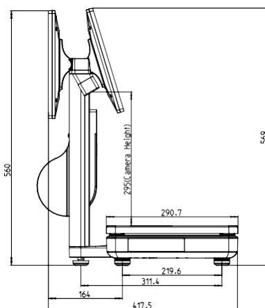
Lateral (tela do cliente de 15,6 polegadas)
