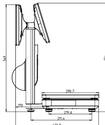
Lateral (tela do cliente de 11,6 polegadas)
