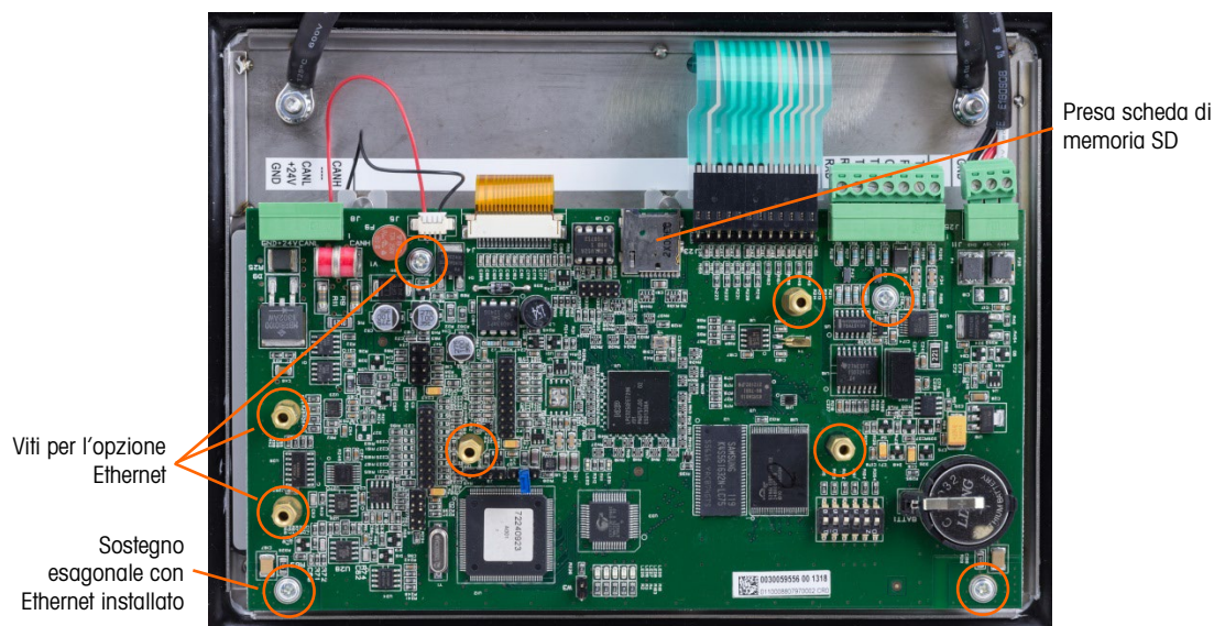
Figura 5-15: Montaggio viti per scheda madre, versione POWERCELL
